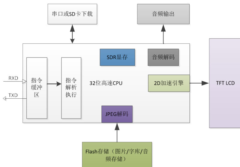
图 10-1 GM 系列串口屏内部结构图
