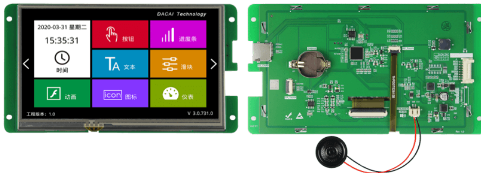
图 1-1 7.0 寸电阻触摸参考图
