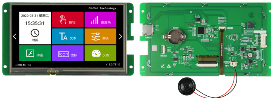
图 1-3 7.0 寸无触摸参考图
