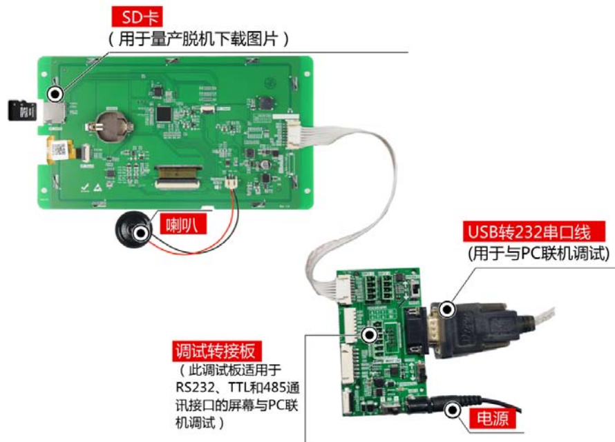
图 1-5 调试工具图
